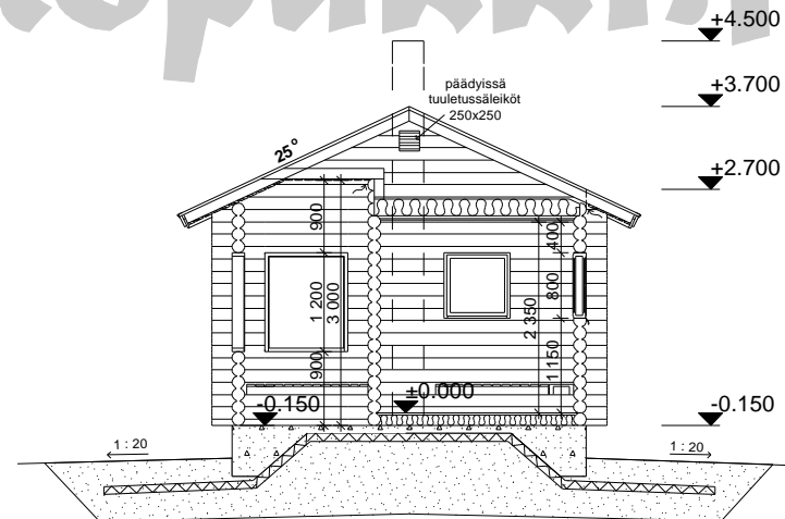
PÄÄTY EDESTÄ VASEMMALLE
