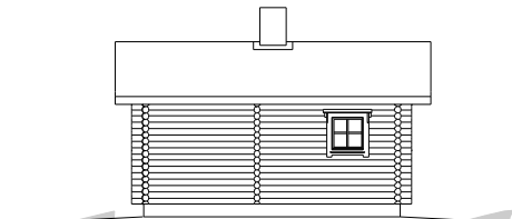
TAKAJULKISIVU
