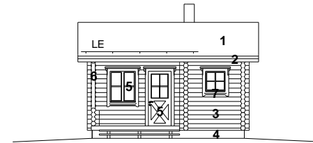
ETUJULKISIVU
