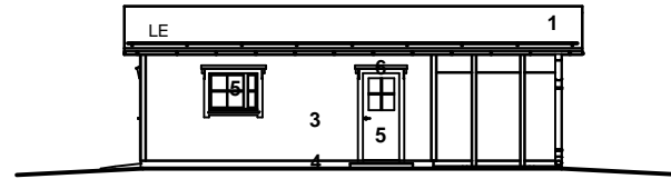
ETUJULKISIVU
